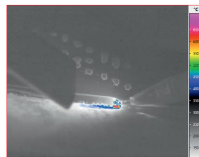
Thermische Analyse beim Laserstrahllöten
