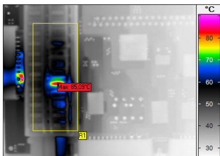
Abb. 2: 5x Digitalzoom eines Wärmebilds mit Sicherungsblock
