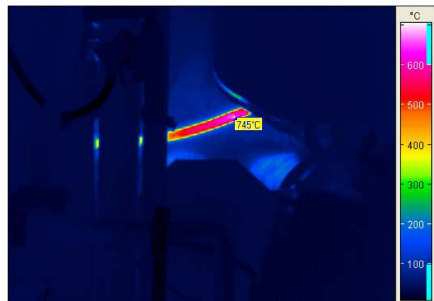
Abb. 3: Thermogramm des Walzgutes zur anschließenden Analyse in einer Spezialsoftware
